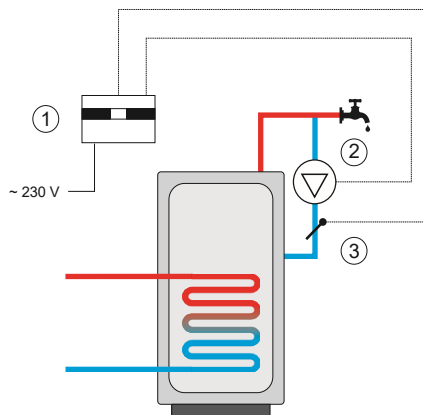
Zīm. 3 Regulatora paraugs savienojums ar karstā ūdens
