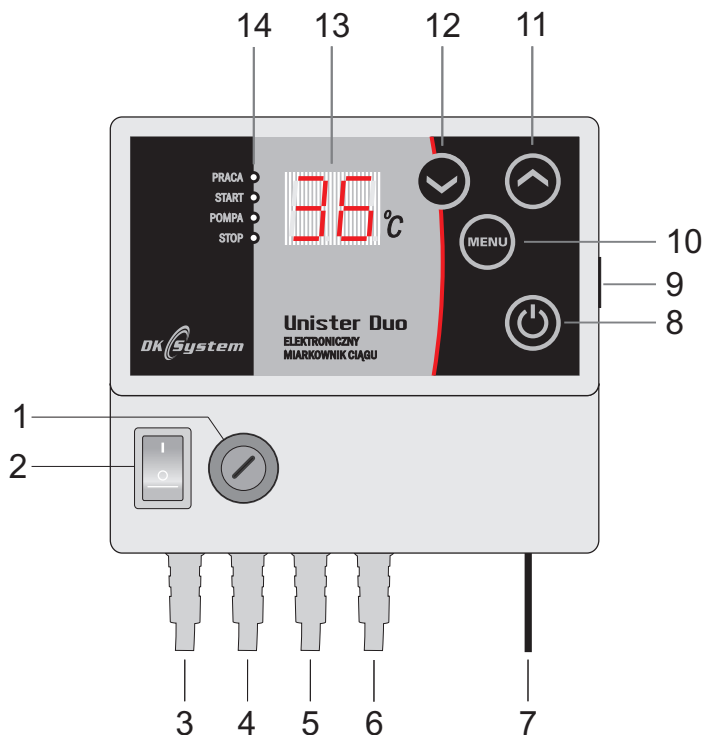
Rys.2 Elementy regulatora
