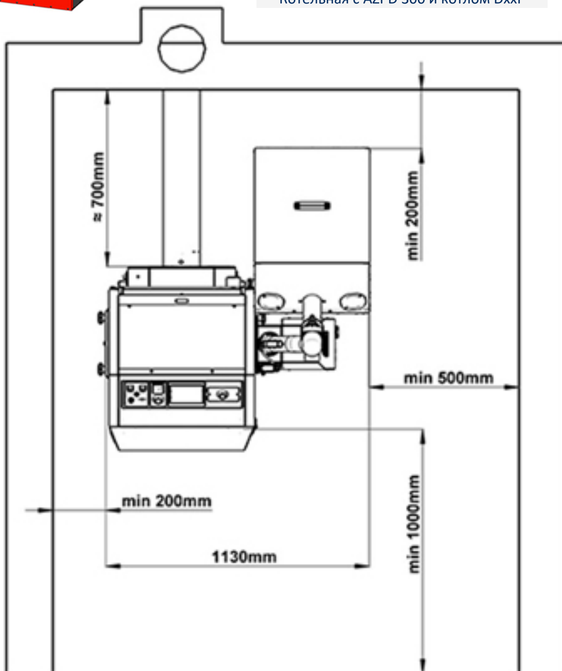
Котельная с AZPD 300 и котлом DxxP
