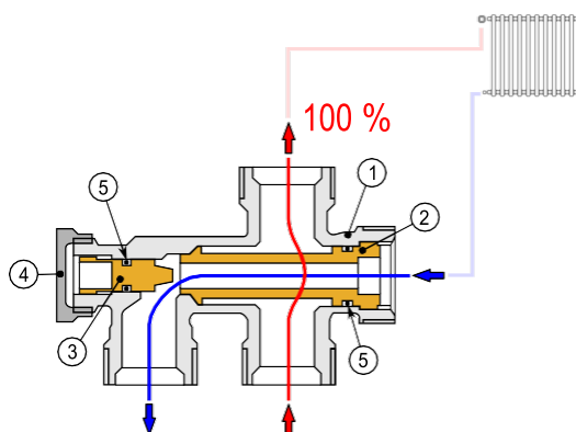
Divu cauruļu sistēma
